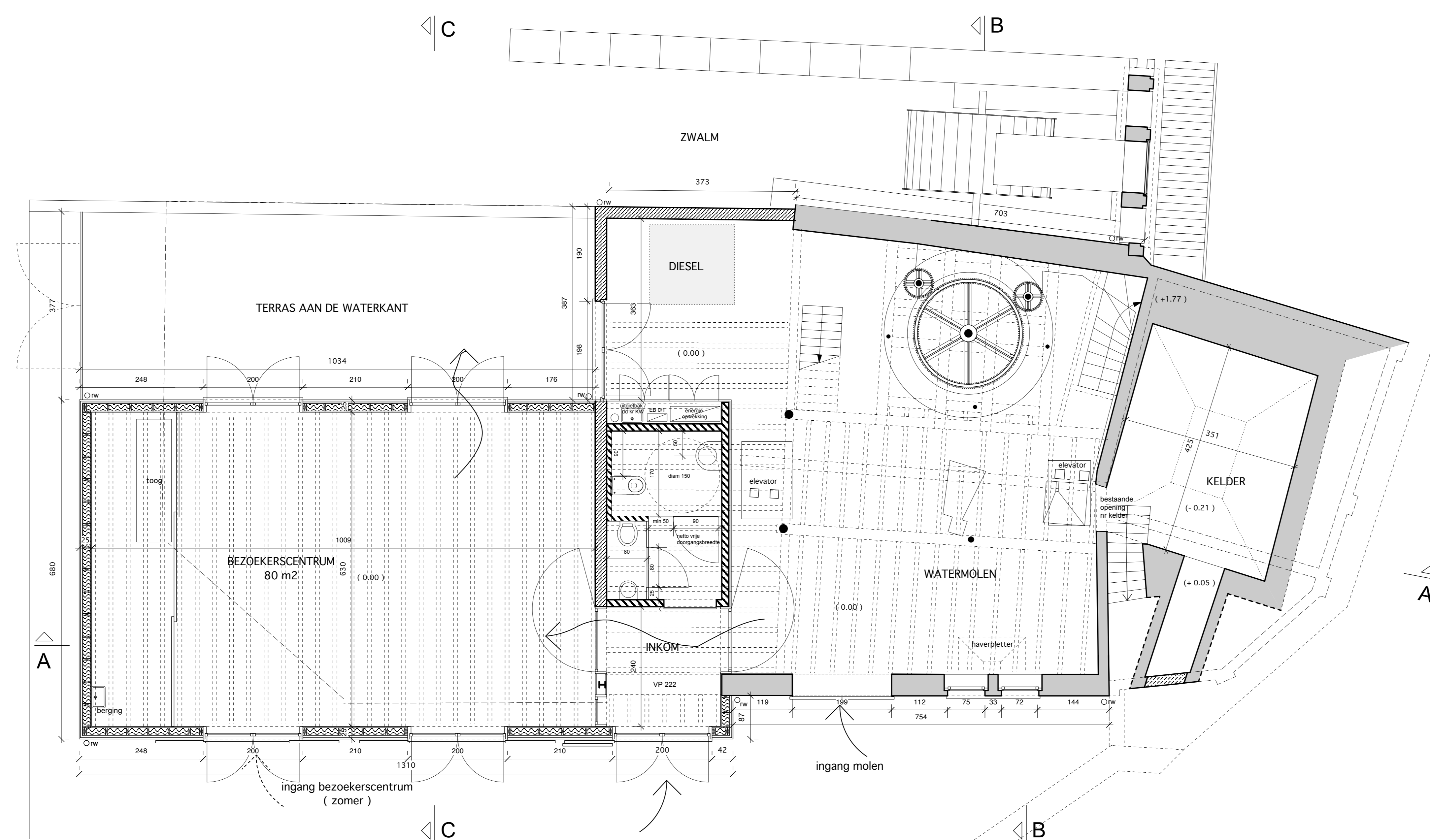
GRONDPLAN nivo 0.00 & -0.21
